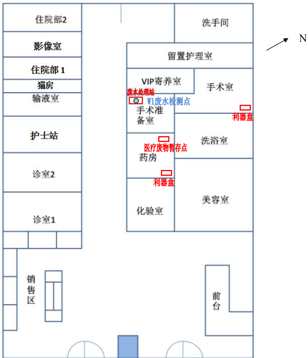
附图 4：项目总平面布置图及医疗废水监测布点图
