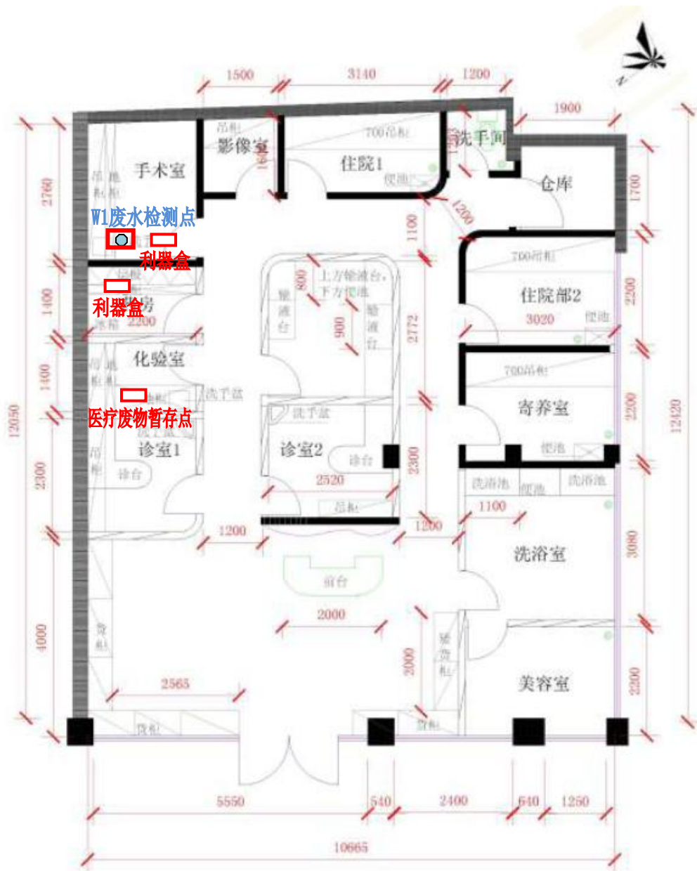
附图 4：项目总平面布置图及医疗废水监测布点图
